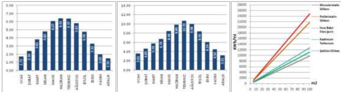
Şekil 5-7. a) Gölbaşı İlçesi Radyasyon Değerleri (KWh/m 2 gün) b) Gölbaşı İlçesi güneş ışığı süreleri (saat) c) Gölbaşı PV tipi-Alan-Üretililecek Enerji (KWh year) 2
